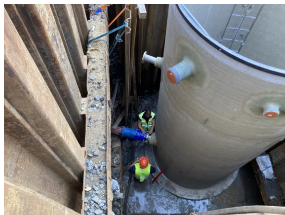
ČSOV 1 – připojení čerpací jímky
