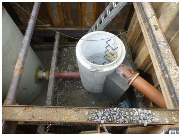
Propojení ČS2 a stoky C1
