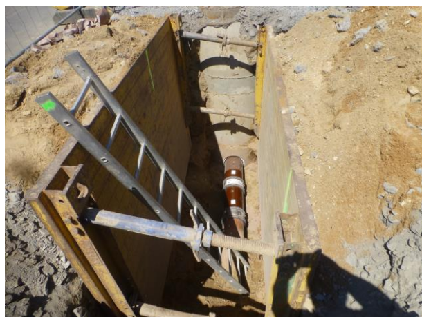
Oprava spoje KT potrubí
