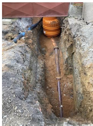
Stoka A – realizace kanalizační přípojky
