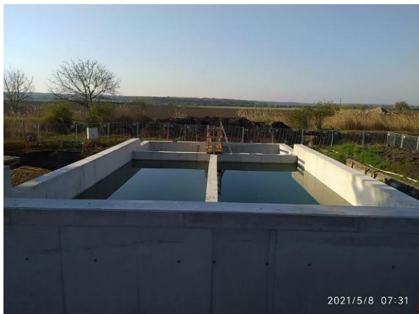
Zkouška těsnosti stěn nádrží ČOV
