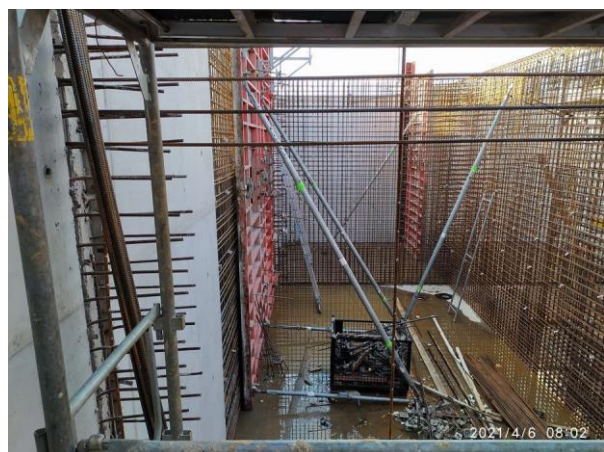
Výztuž vnitř.stěn nádrží ČOV
